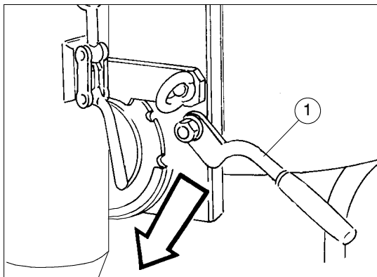
1 Заслонка материала
