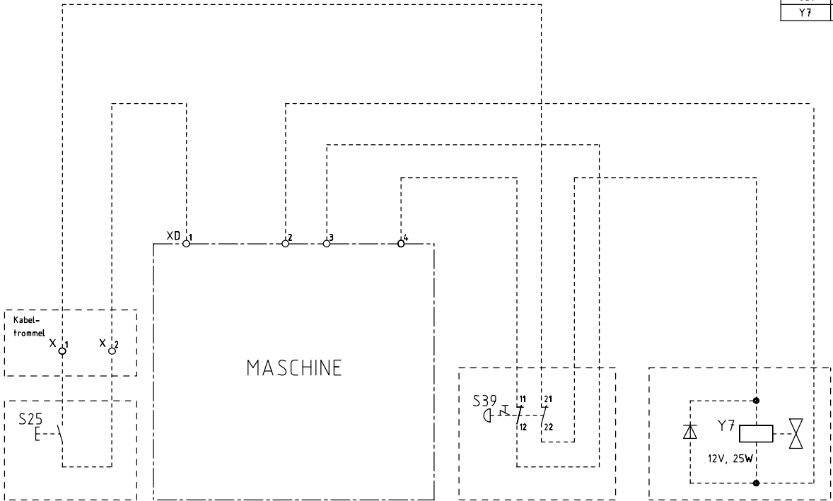
KABELFERNSTEUERUNG
